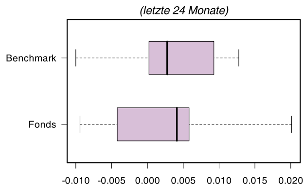
Boxplot der monatlichen Returns
